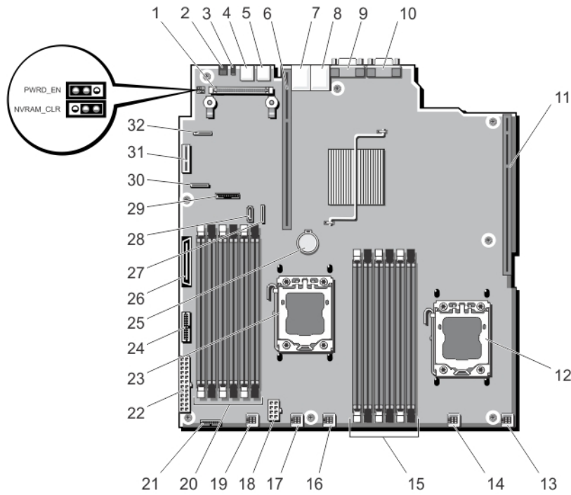
图 40: 系统板跳线和连接器
