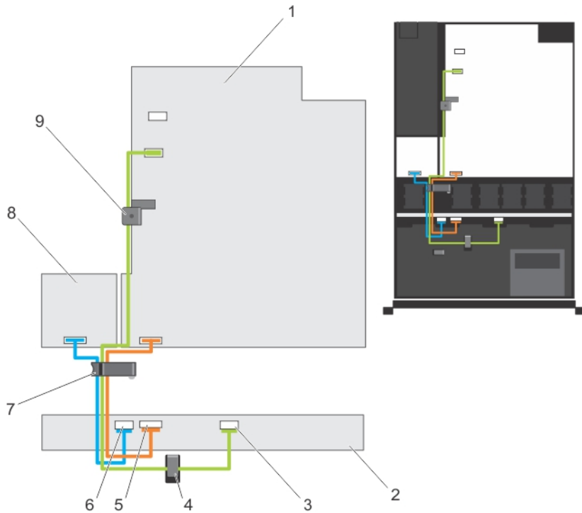
图 34: 布线图 — 四硬盘驱动器背板
