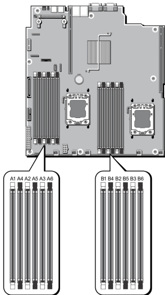
图 11: 内存插槽位置
