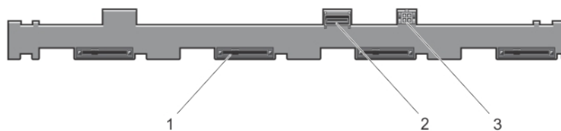
图 31: 四硬盘驱动器背板的正面视图
