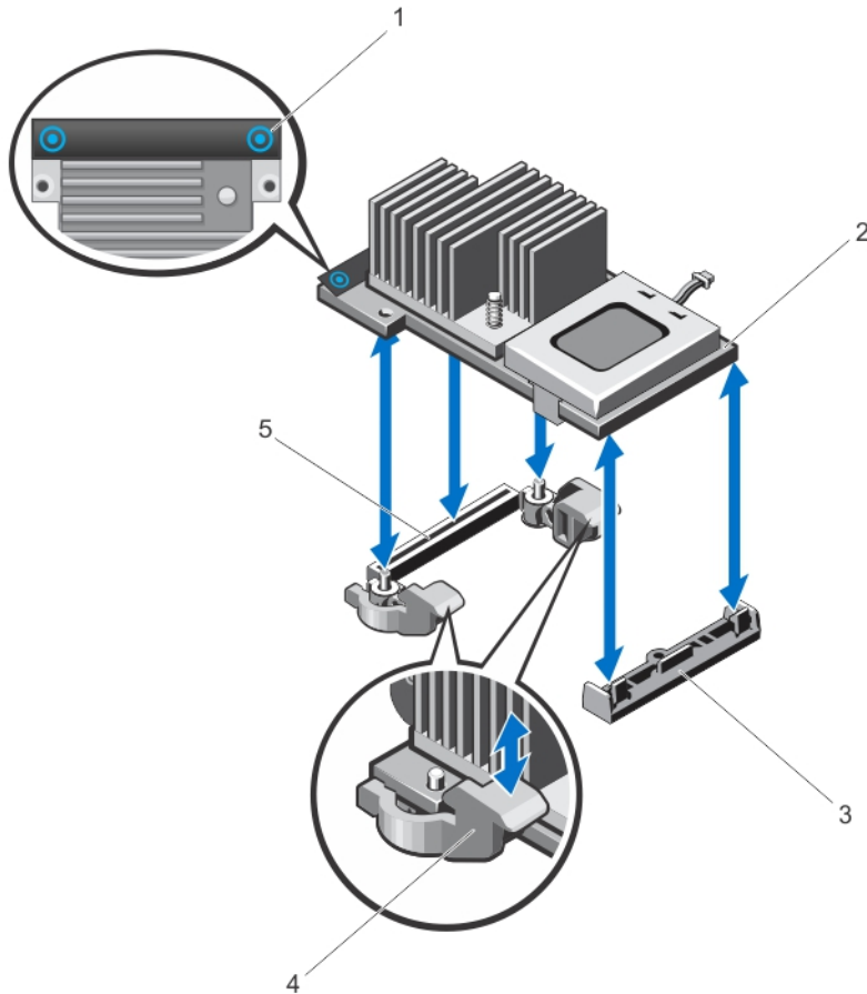
图 26: 卸下和安装集成存储控制器卡
