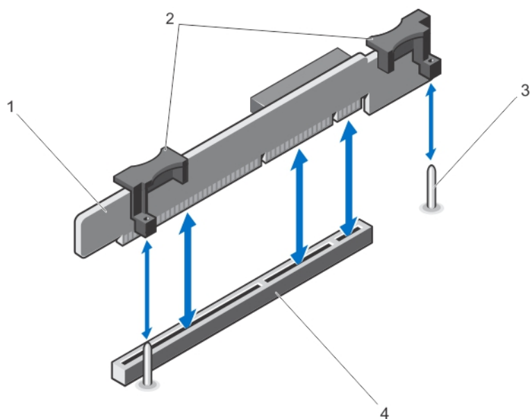
图 21: 卸下和安装扩充卡提升板 1
