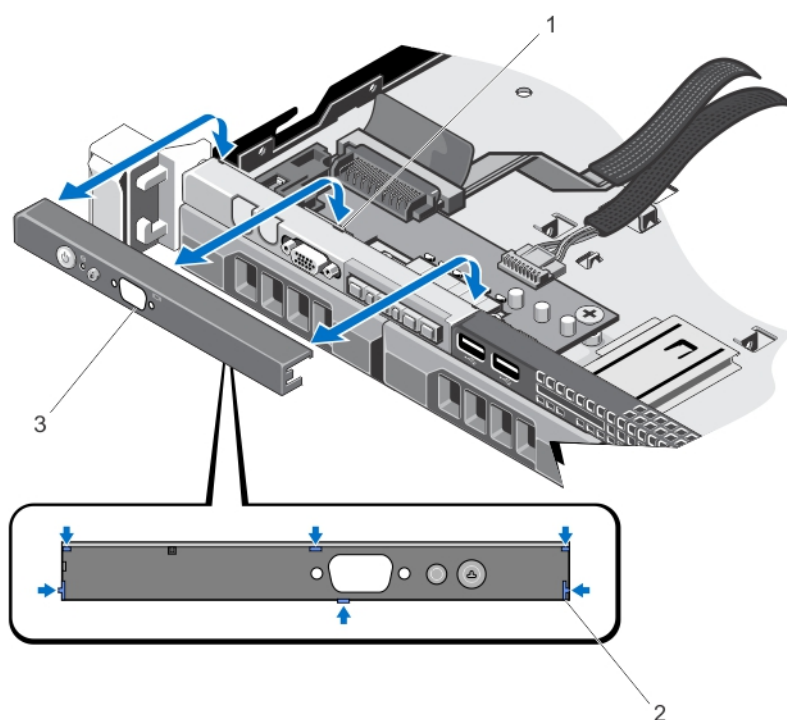
图 35: 卸下和安装控制面板
