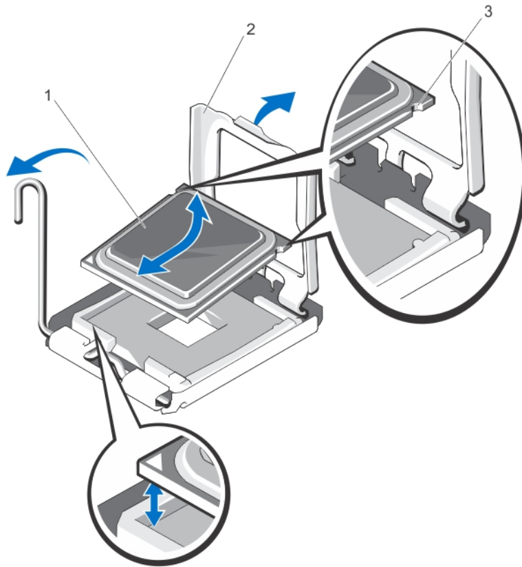
图 28: 卸下和安装处理器
