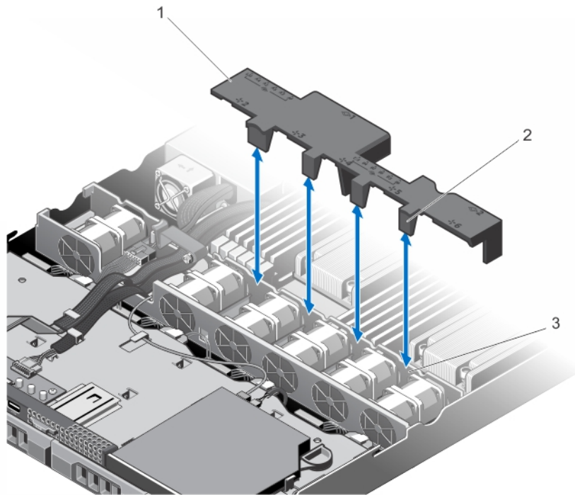
图 10: 卸下和安装冷却导流罩
