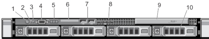
图 1: 前面板部件和指示灯
