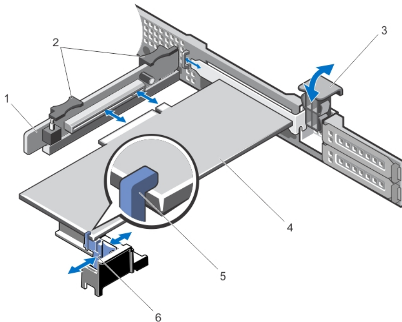
图 20: 在扩充卡提升板 2 中卸下和安装扩充卡
