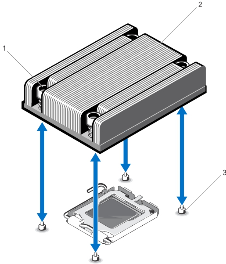
图 27: 卸下和安装处理器散热片
