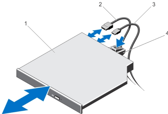
图 16: 卸下和安装光盘驱动器
