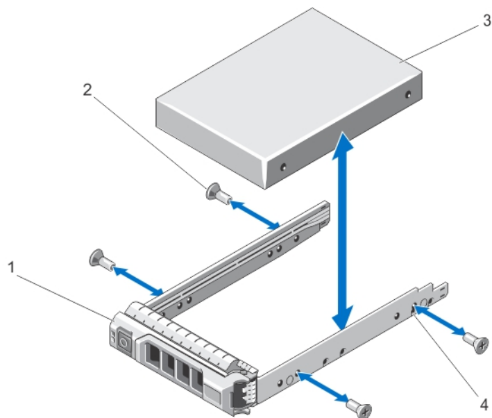
图 15: 在硬盘驱动器托盘中卸下和安装热插拔硬盘驱动器
