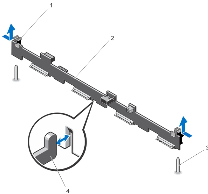
图 33: 卸下和安装四硬盘驱动器背板
