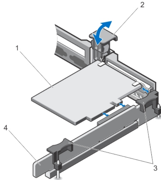
图 19: 在扩充卡提升板 1 中卸下和安装扩充卡
