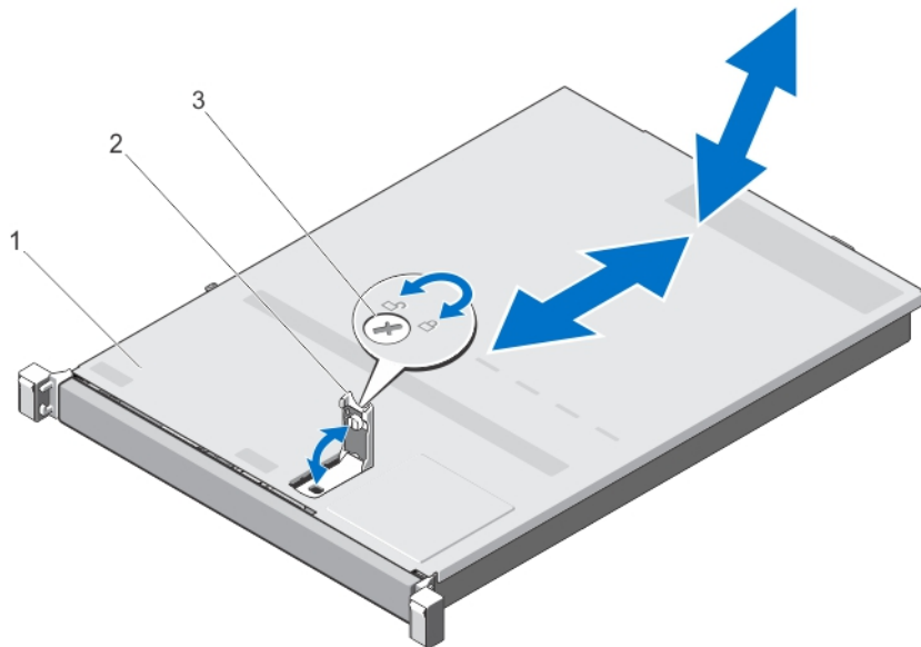
图 8: 打开与合上系统护盖
