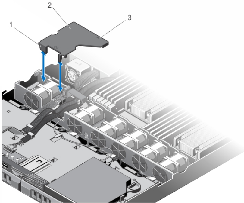
图 37: 卸下和安装 PDB 导流罩
