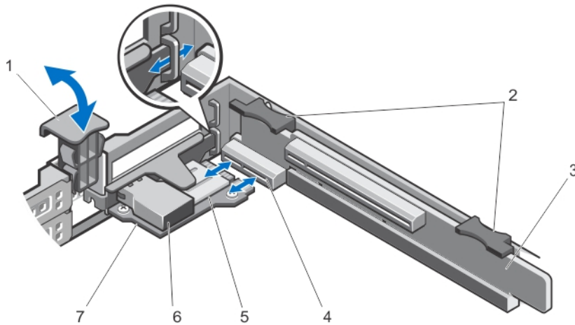
图 23: 卸下和安装 iDRAC 端口卡
