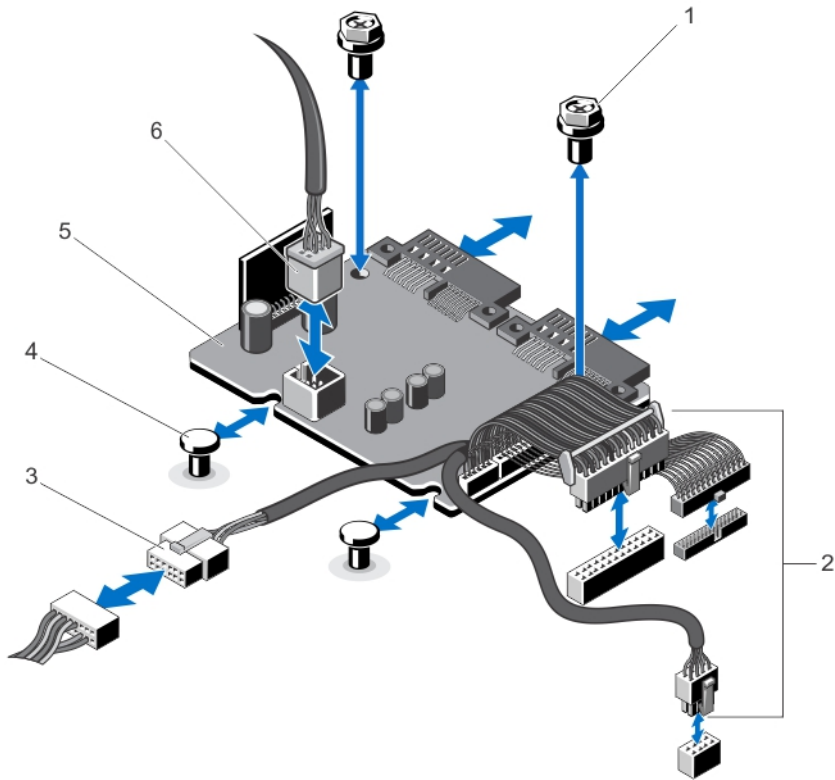
图 38: 卸下和安装配电板
