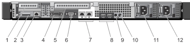
图 4: 背面板部件和指示灯
