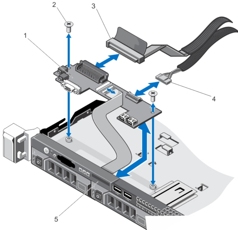
图 36: 卸下和安装控制面板模块
